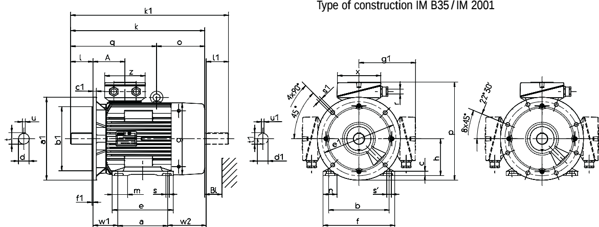
Type of construction IM B35/IM 2001
