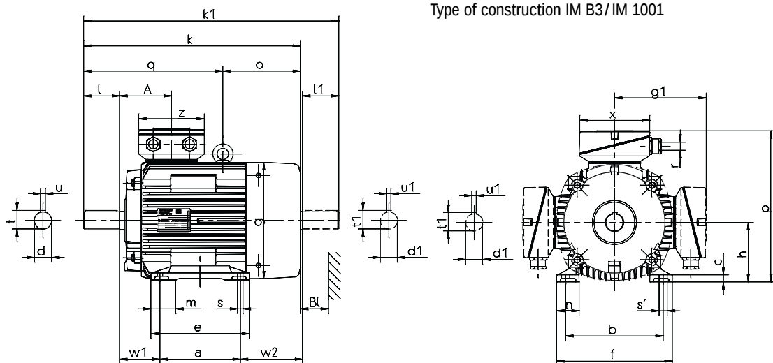
Type of construction IM B3/IM 1001
