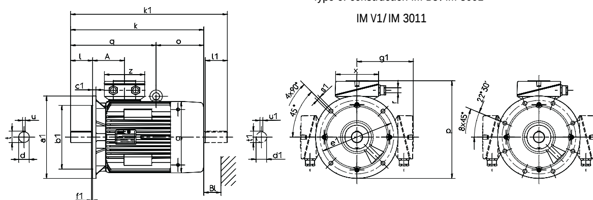
Type of construction IM B5/IM 3001
