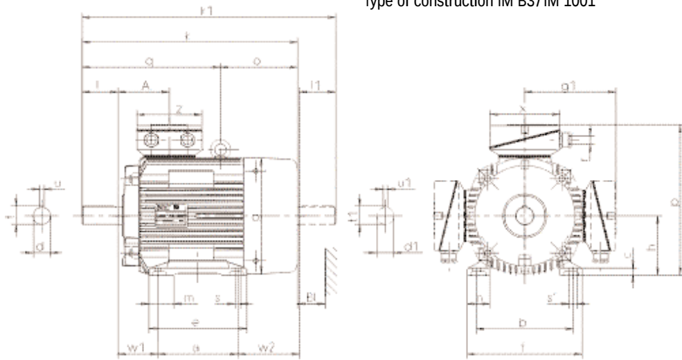
Type of construction IM B3/IM 1001
